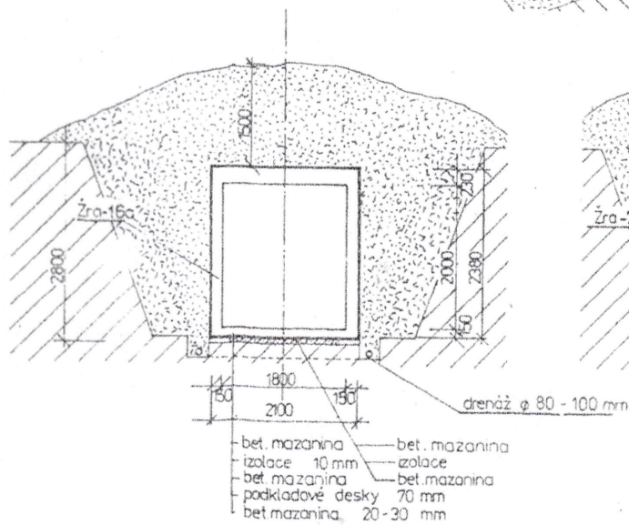
Řez 3-3'
