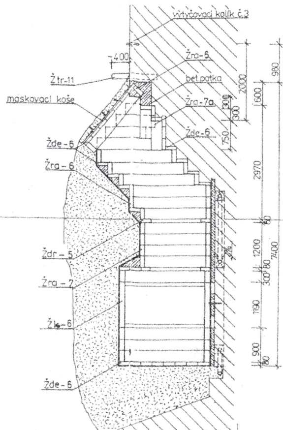
Řez 4-4'
