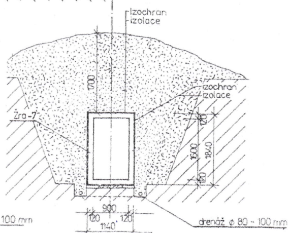
Řez 4-4'
